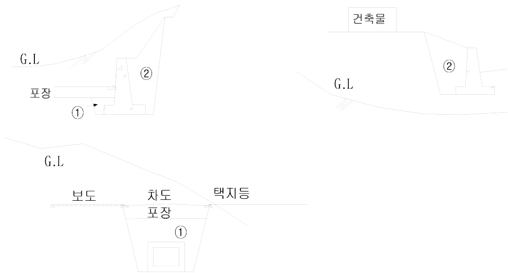
부록 1 그림 2-1 구조물 되메우기
