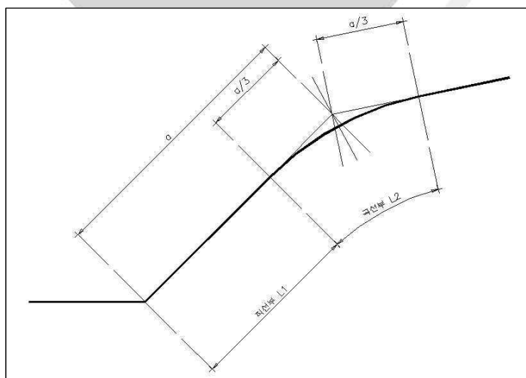
<그림 4.6-1> 사면 라운딩 방법의 모식도
