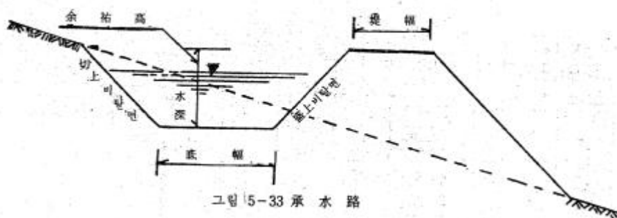
<그림 4.4-1> 승수로
