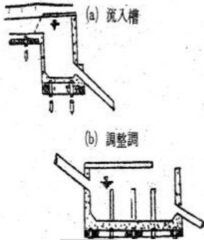
<그림 4.4-2> 조정수조
