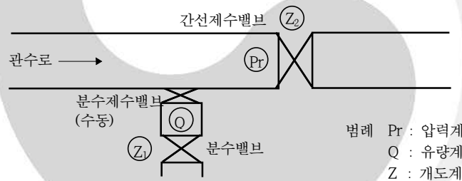
<그림 4.2-5> 관수로 분수공(폐쇄형)시설 개략도
