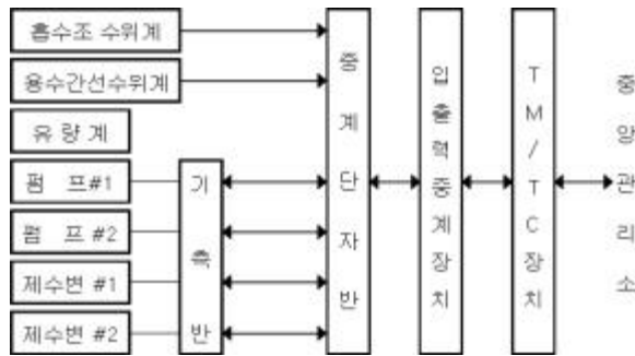
<그림 4.2-4> 양수장 장치도
