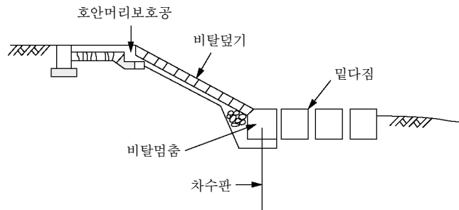
그림 4.2-1 호안의 구조
