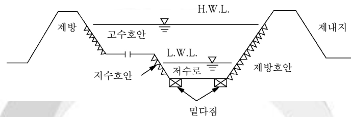
그림 4.4-1 호안의 설치위치별 종류
