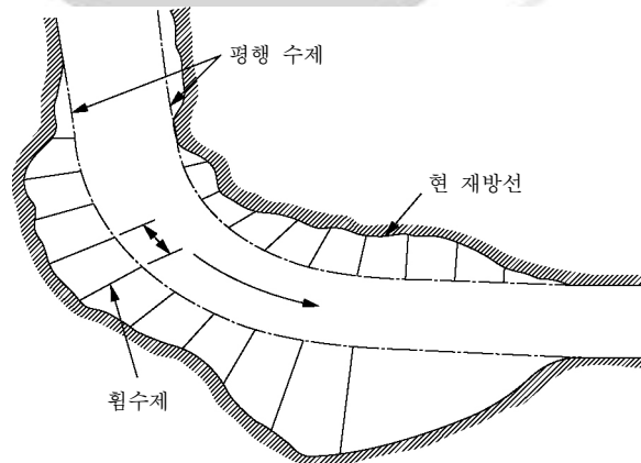
그림 4.8-1 수제 일반도
