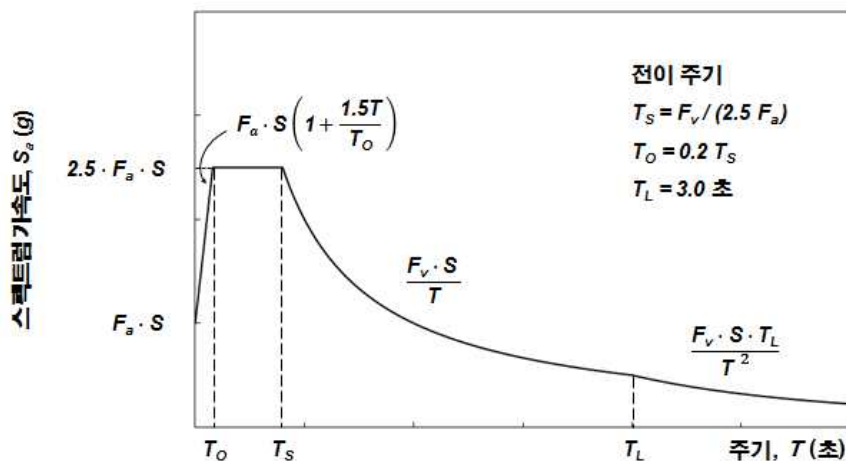
그림 4.2-2 가속도표준설계응답스펙트럼 (토사지반)
