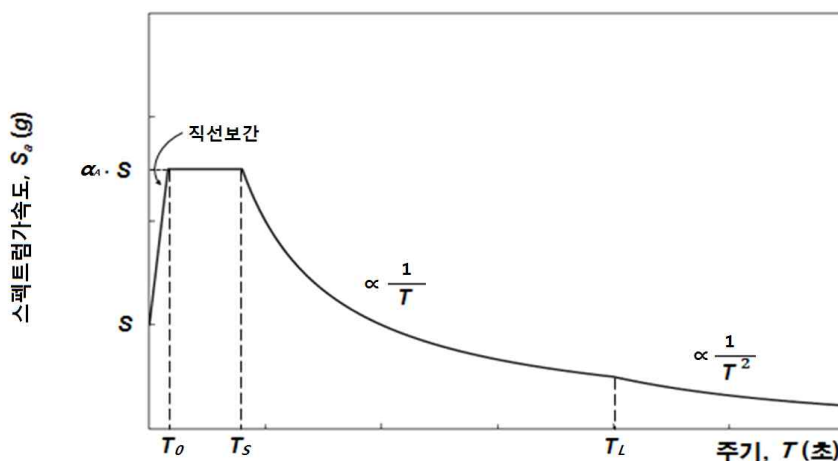
그림 4.2-1 가속도표준설계응답스펙트럼 (암반지반)
