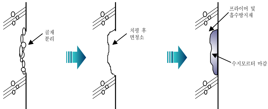
그림 3.1-6 골재분리 부분 보수
