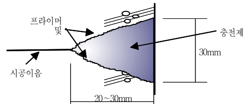
(a) 시공이음 보수
