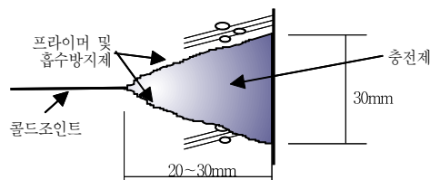
(b) 콜드조인트 보수
