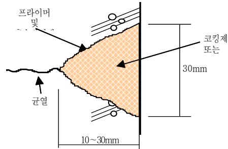
그림 3.1-2 균열보수(충전제 메움)
