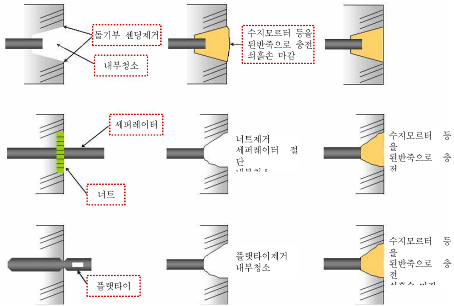
그림 3.1-1 폼타이 및 플랫타이 제거 및 구멍 보수
