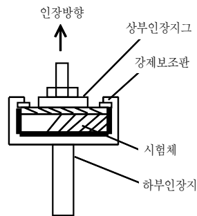
(a) 시험편과 상부 인장지그 결합도
