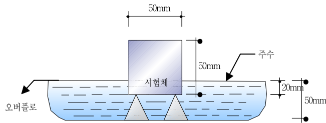
그림 3.6-1 흡수시험방법
