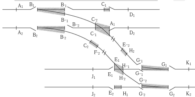
그림 3.3-3 건넘선의 장대레일 재설정
