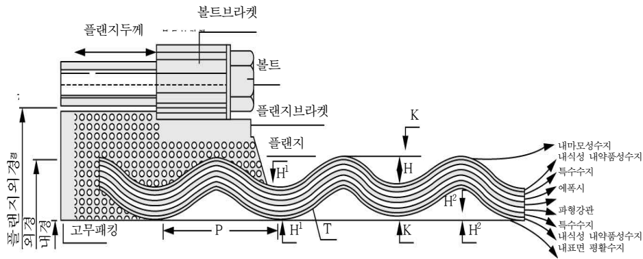
그림 2.4-3 수지파형강관 단면도(평활형)
